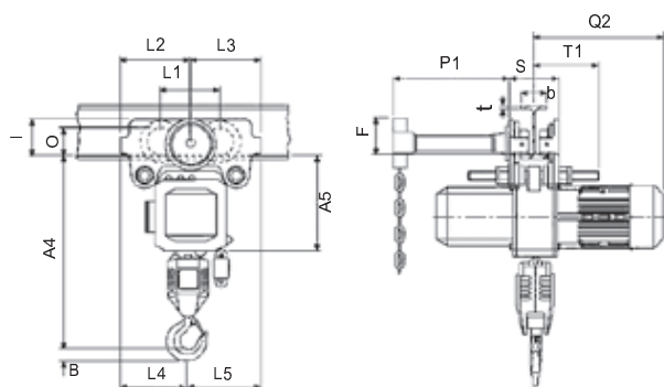
Modelo CPEF com trole mecânico 7500 kg
