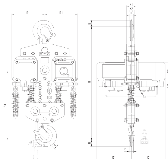
Modelo CPA ATEX - suspensão por gancho 10t - 4 ramaís
