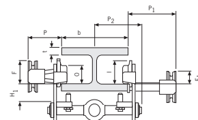
Modelo HTP/HTG ATEX com dispositivo de travamento 0,5 / 5t
