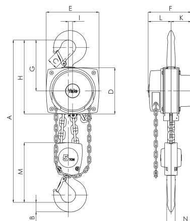
Modelo Yalelift 360 ATEX, 5t, 2 ramais de corrente
