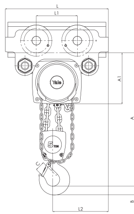
Modelo Yalelift ITP/ITG ATEX, 5t, 2 ramais de corrente
