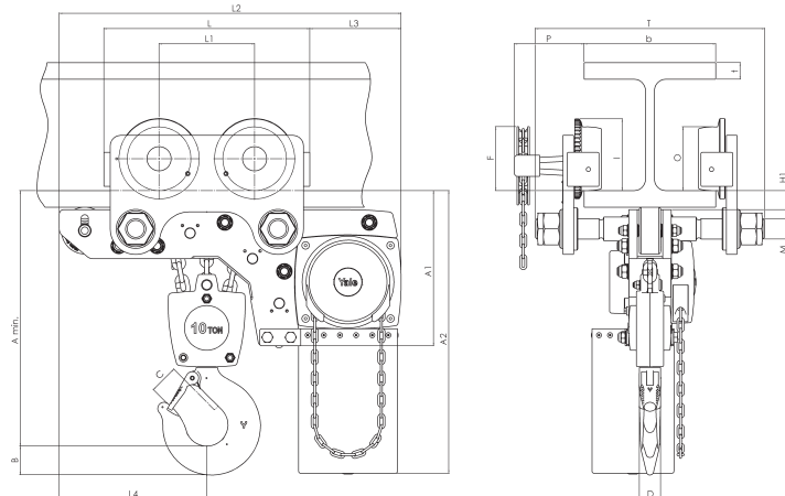
Modelo Yalelift LHG ATEX, 10t, 3 ramais de corrente
