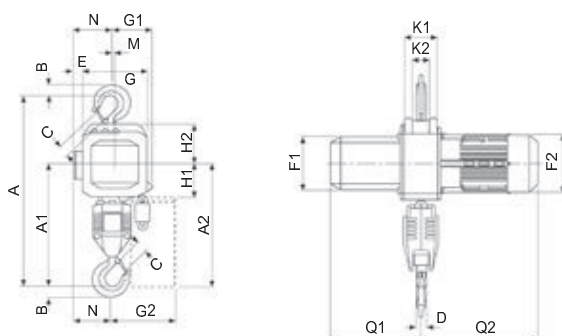
Modelo CPEF com suspensão por gancho 4000 Kg e 5000 kg (2 ramaís de corrente)
