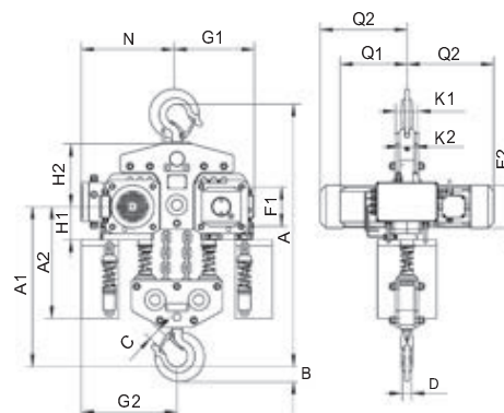
Modelo CPEF com suspensão por gancho 10000 kg (4 ramaís de corrente)
