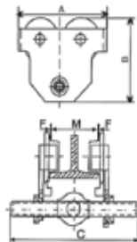
Especificações técnicas - GCTY - MANUAL
