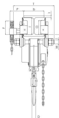
Modelo Yalelift ITG ATEX, 0,5/3t, 1 ramal de corrente
