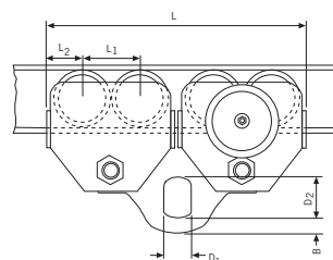
Modelo HTG ATEX, 20t
