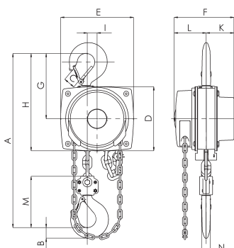
Modelo Yalelift 360 500 - 3.000 kg, um ramal
