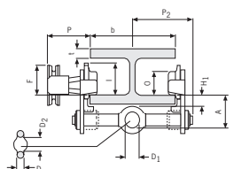
Modelo HTP/HTG ATEX, 0,5 / 5t
