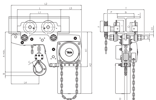
Modelo Yalelift LHG ATEX, 0,5/3t, 1 ramal de corrente
