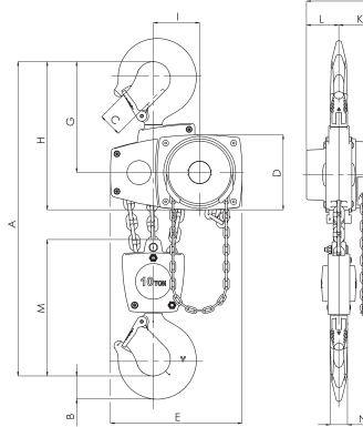
Modelo Yalelift 360 10.000 kg, três ramais
