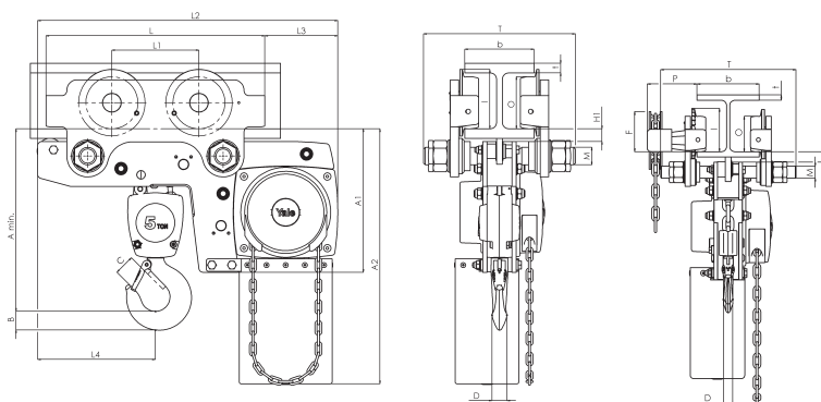
Modelo Yalelift LHP/LHG ATEX, 5t, 2 ramais de corrente
