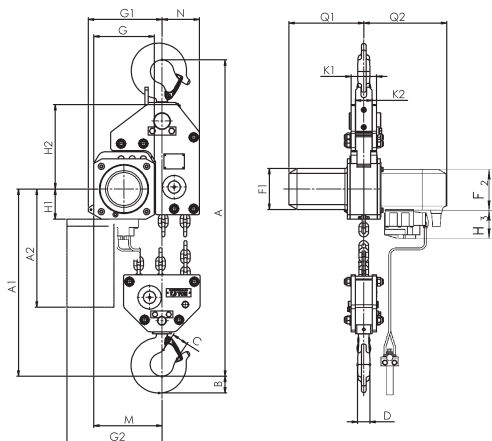
Modelo CPA ATEX - suspensão por gancho 7,5t - 3 ramaís
