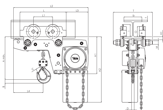
Modelo Yalelift LHP ATEX, 0,5/3t, 1 ramal de corrente
