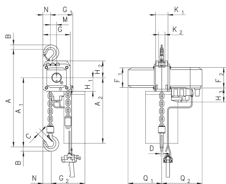
Modelo CPA ATEX - suspensão por gancho 2/3t - 1 ramal
