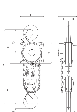
Modelo Yalelift 360 5.000 kg, dois ramais
