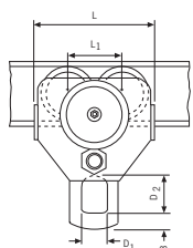
Modelo HTG ATEX, 10t
