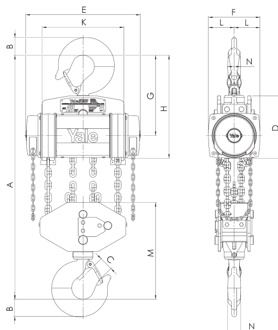
Modelo Yalelift 360 ATEX, 20t, 6 ramais de corrente
