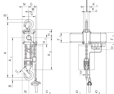
Modelo CPA ATEX - suspensão por gancho 4/5t - 2 ramaís
