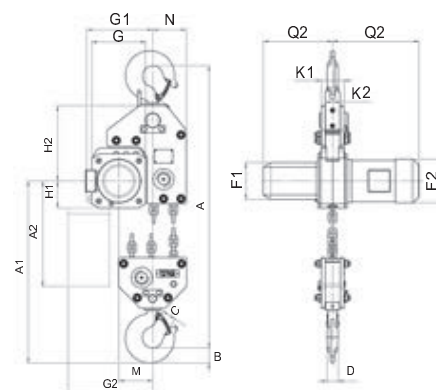
Modelo CPEF com suspensão por gancho 10000 kg (4 ramaís de corrente)
