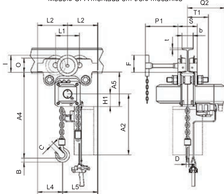
Modelo CPA montada em trole mecânico
