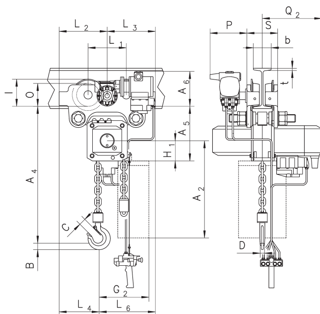
Modelo CPA ATEX - integrado com trole pneumático
