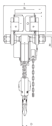
Modelo Yalelift ITP/ITG ATEX, 5t, 2 ramais de corrente
