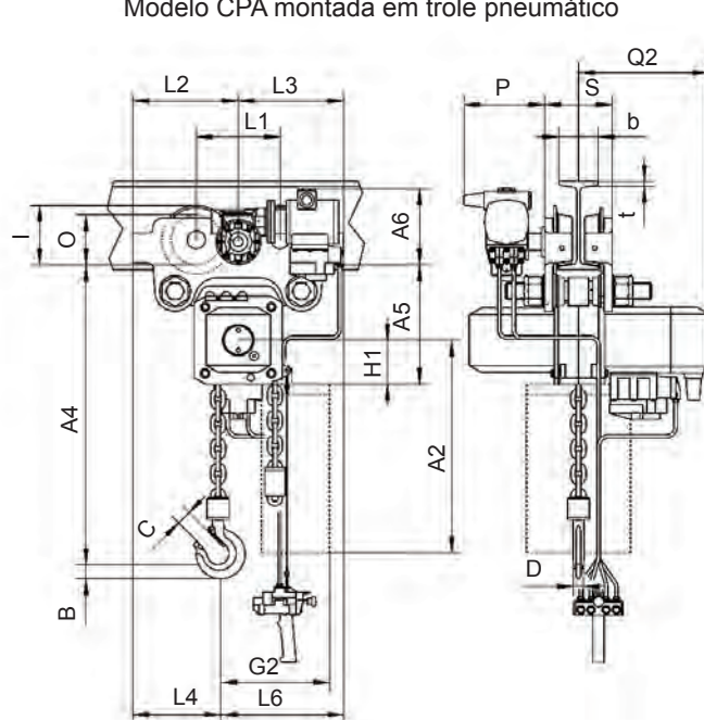
Modelo CPA montada em trole pneumático
