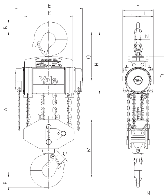
Modelo Yalelift 360 ATEX, 20t, 6 ramos de corrente
