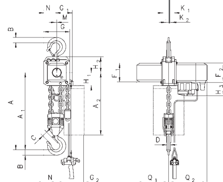
Modelo CPA ATEX - suspensão por gancho 4/5t - 2 ramais
