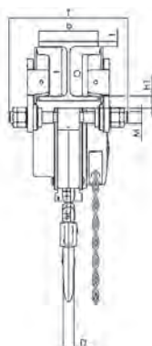
Modelo Yalelift ITP ATEX, 0,5/3t, 1 ramal de corrente
