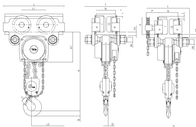
Modelo Yalelift ITP/ITG - troles manual e mecânico 5.000 kg, dois ramais
