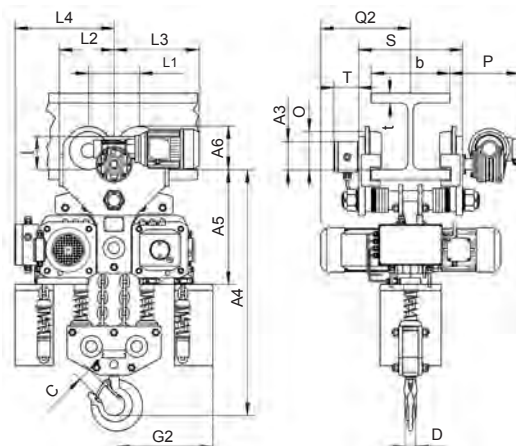
Modelo CPEF com trole elétrico 10000 kg
