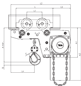
Modelo Yalelift LHP ATEX, 0,5/3t, 1 ramal de corrente
