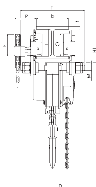
Modelo Yalelift ITG ATEX, 0,5/3t, 1 ramal de corrente
