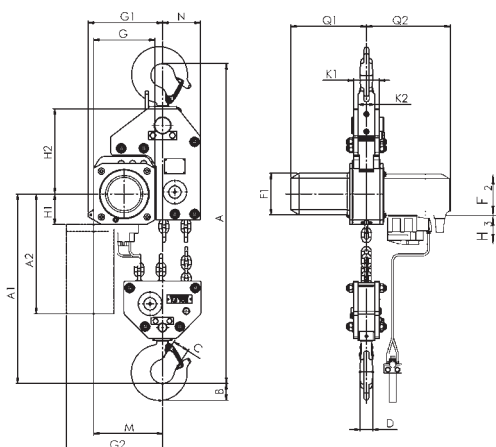
Modelo CPA ATEX - suspensão por gancho 7,5t - 3 ramais
