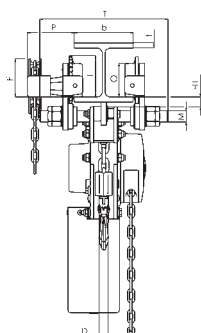
Modelo Yalelift LHG ATEX, 0,5/3t, 1 ramal de corrente
