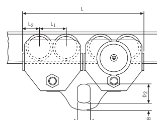
Modelo HTG ATEX, 20t
