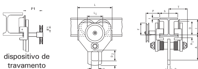
Modelo HTG ATEX, 10t
