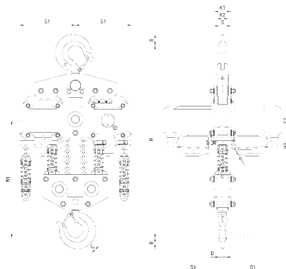
Modelo CPA ATEX - suspensão por gancho 10t - 4 ramais
