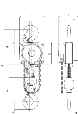
Modelo Yalelift 360 5.000 kg, dois ramais
