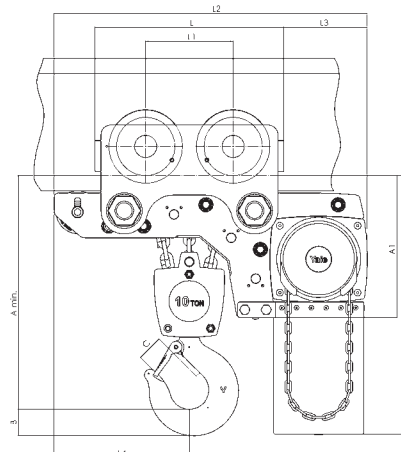
Modelo Yalelift LHG ATEX, 10t, 3 ramais de corrente
