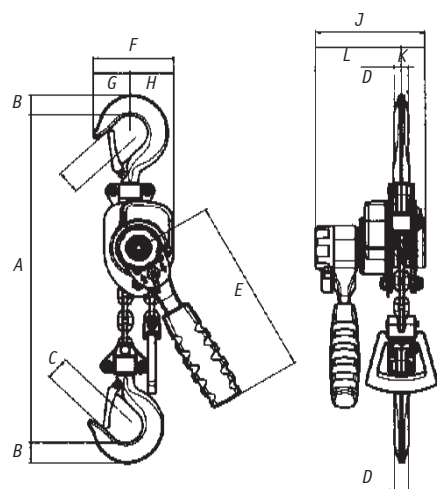
Modelo GCTY Manual
