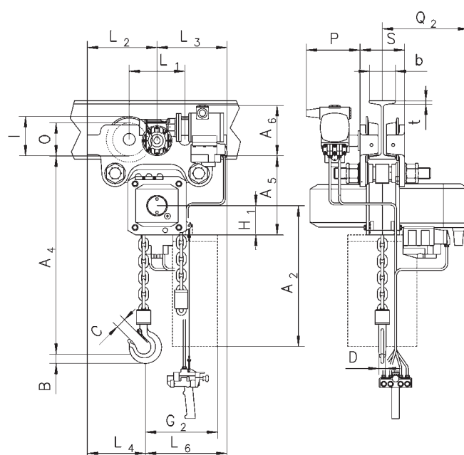
Modelo CPA ATEX - integrado com trole pneumático
