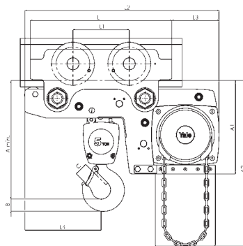
Modelo Yalelift LHP/LHG ATEX, 5t, 2 ramais de corrente
