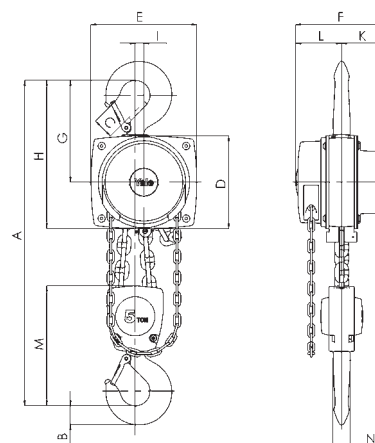
Modelo Yalelift 360 ATEX, 5t, 2 ramos de corrente
