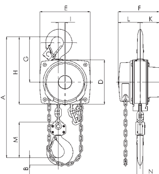
Modelo Yalelift 360 500 - 3.000 kg, um ramal
