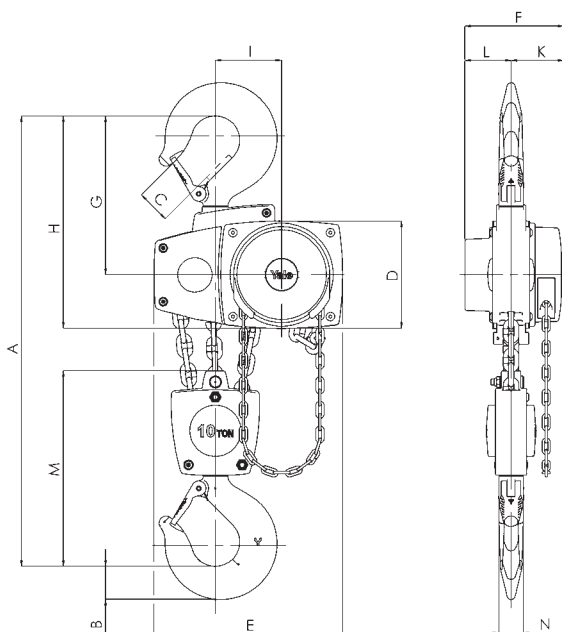
Modelo Yalelift 360 ATEX, 10t, 3 ramos de corrente
